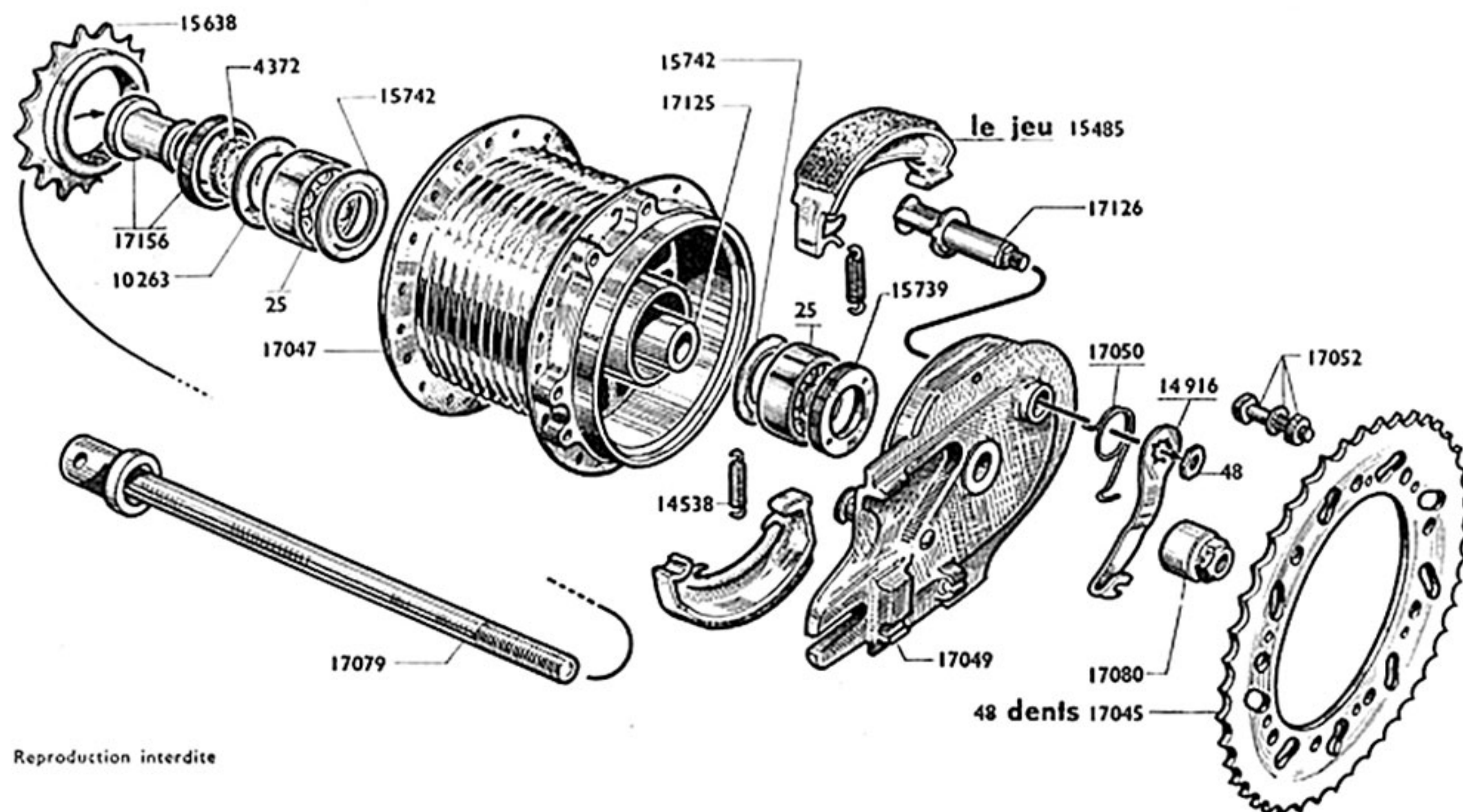
moyeu arrière complet 17044
