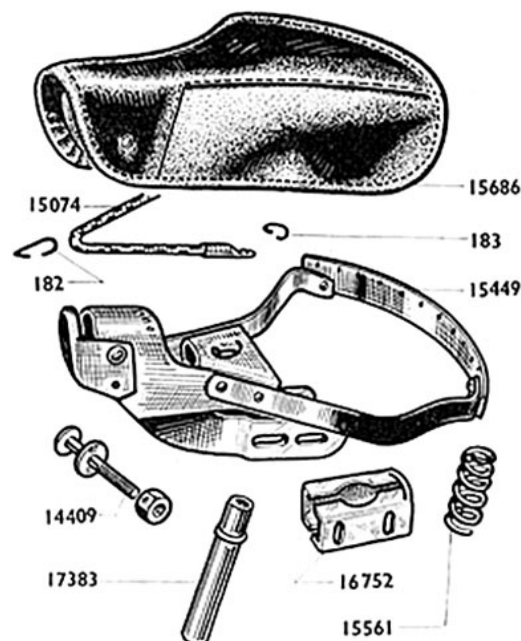
Selle complète 16798 Reydel
