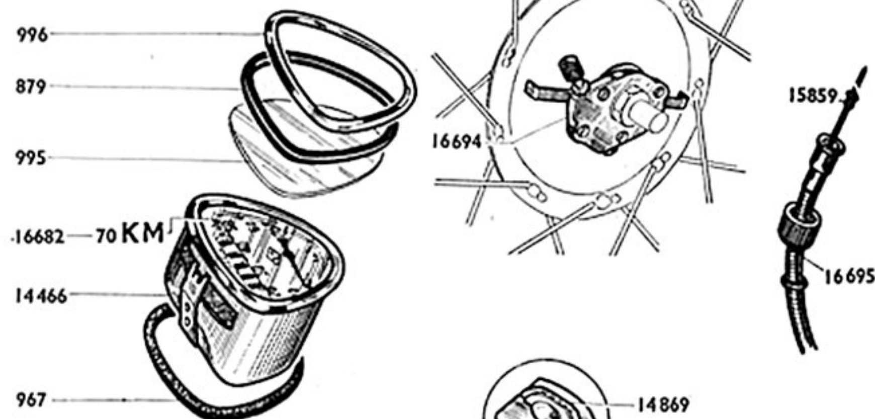
Compteur complet E D 15856
